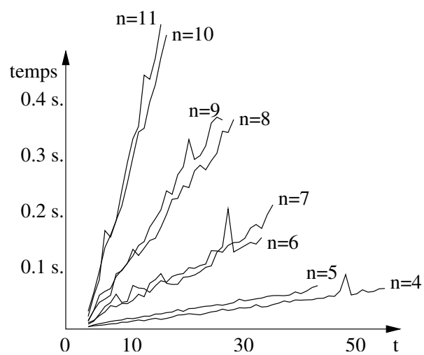
FIG. IV.3 – Performance en grande dimension
